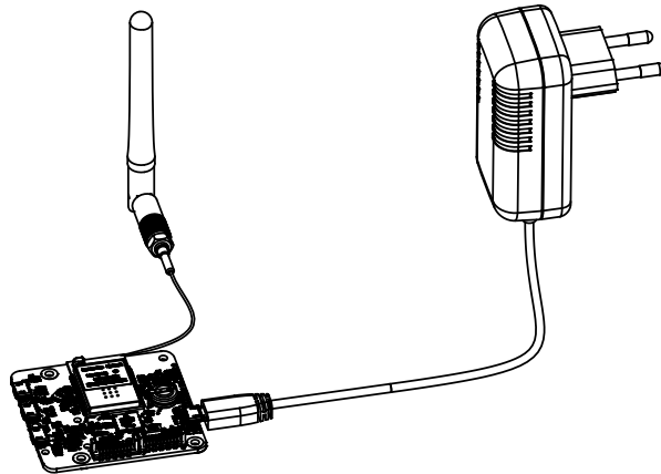
Le YoctoHub-Wireless-SR peut être alimenté par un chargeur USB
