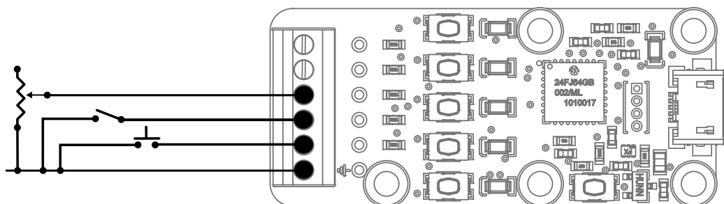
Câblage d'un potentiomètre, d'un interrupteur et d'un bouton poussoir, en masse commune.
