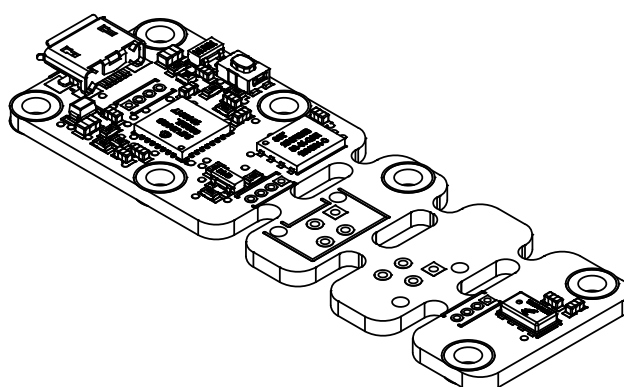
Le module Yocto-Altimeter
