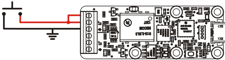
Câblage avec pull-up: la tension haute est fournie par le Yocto-PWM-Rx, le générateur de signal se contente de tirer le signal à la terre.
