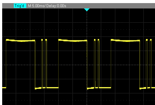
Signal périodique complexe
