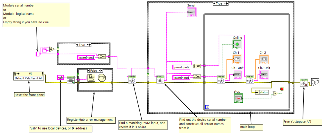
Exemple d'utilisation du Yocto-PWM-Rx dans LabVIEW
