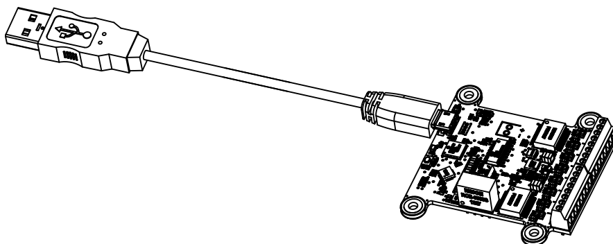
Vous devez raccorder votre module Yocto-Maxi-IO-V2 à l'aide d'un cable USB 2.0 de type A - micro B
