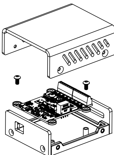
Vous pouvez installer votre Yocto-Maxi-IO-V2 dans un boîtier optionnel.
