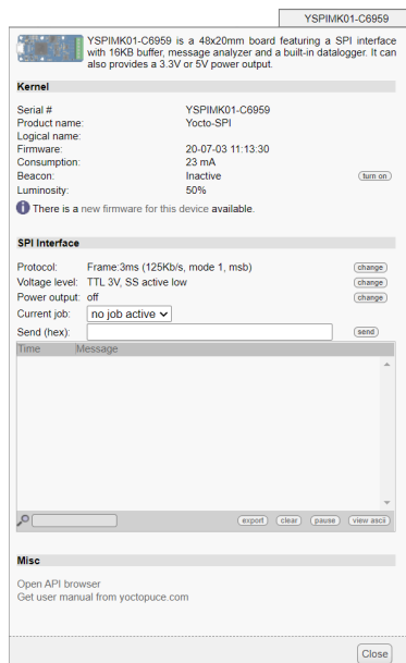
Propriétés du module Yocto-SPI.
