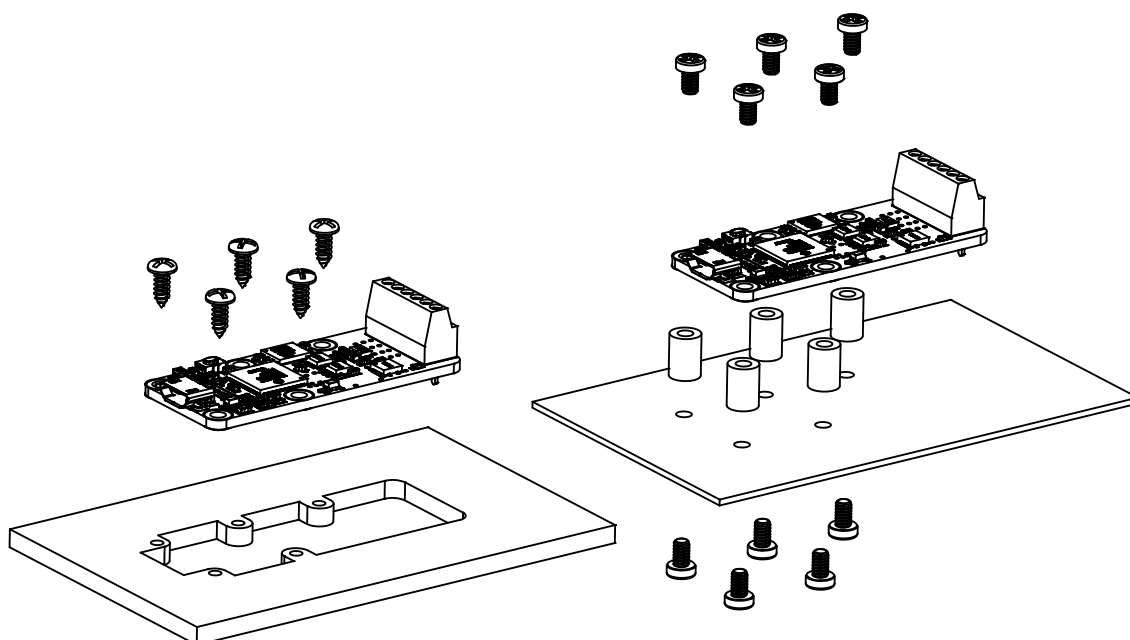
Exemples de montage sur un support.
