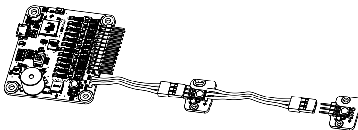
Exemple de câblage des modules LED à l'aide de câbles de servos
