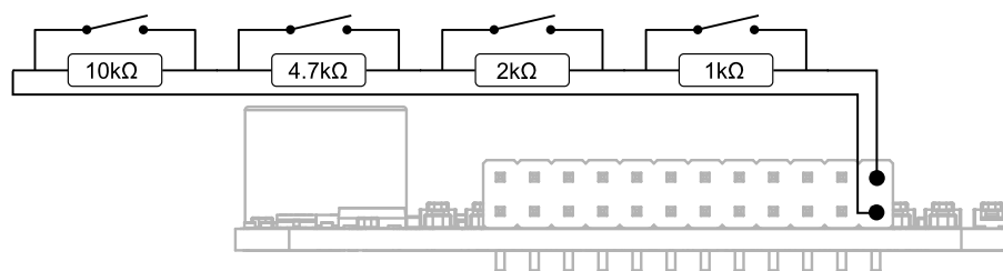
Multiplexage d'entrées on/off sur une entrée analogique
