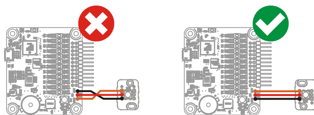
Attention à la polarité et au sens des modules LED, chacun a une entrée et une sortie.
