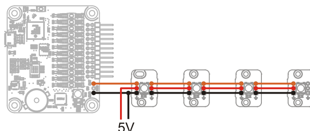
Câblage avec une alimentation externe
