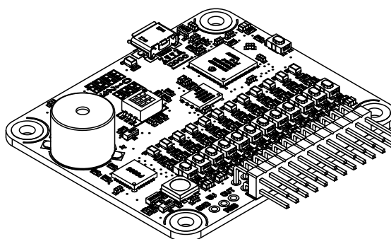
Le module Yocto-MaxiKnob
