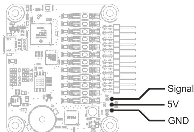
Le module Yocto-MaxiKnob dispose d'une sortie pour piloter des LED supplémentaires
