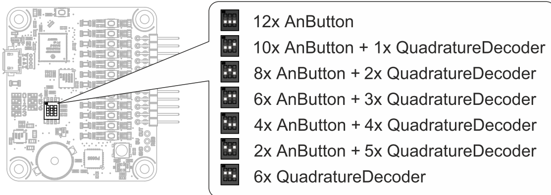
Configuration des micro-interrupteurs
