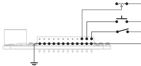
Exemples de connexion d'interrupteur, boutons poussoir, potentiomètres..
