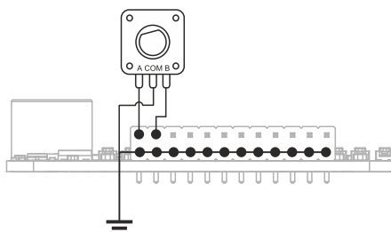
Exemple de connexion d'un encodeur en quadrature
