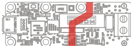
Barrière d'isolation de sécurité du module Yocto-Amp
