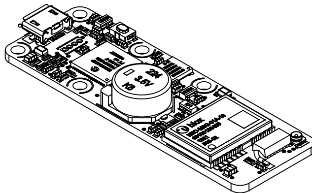
The Yocto-GPS-V2 module
