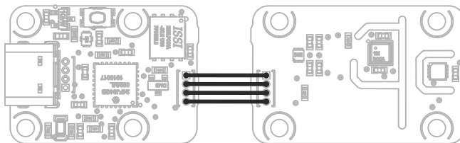
Câblage des sous modules une fois ceux-ci séparés.
