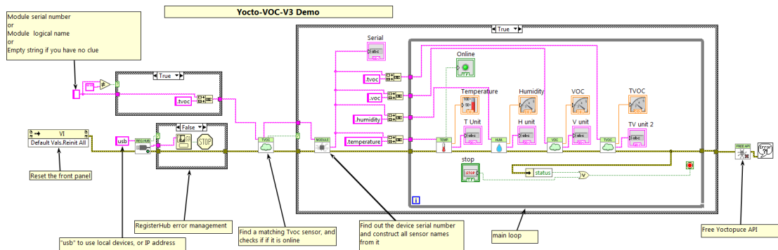
Exemple d'utilisation du Yocto-VOC-V4-C dans LabVIEW
