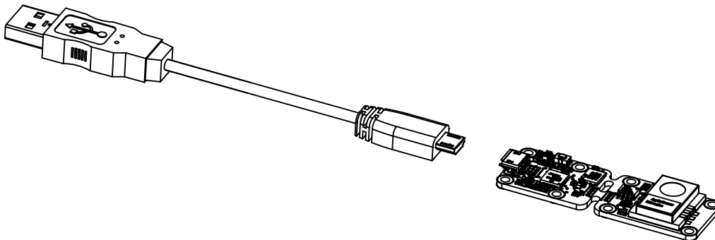
Vous devez raccorder votre module Yocto-VOC-V2 à l'aide d'un câble USB 2.0 de type A - micro B
