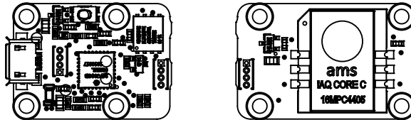
Le module Yocto-VOC-V2 est conçu pour pouvoir être séparé en deux parties...
