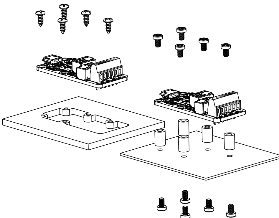
Exemples de montage sur un support.
