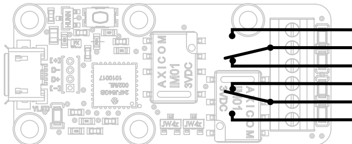
Câblage du relais à l'intérieur du module.
