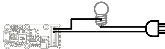
Commander une ampoule à l'aide de votre module Yocto-Relay.
