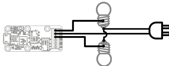
Commander deux ampoules en alternance à l'aide de votre module Yocto-Relay.
