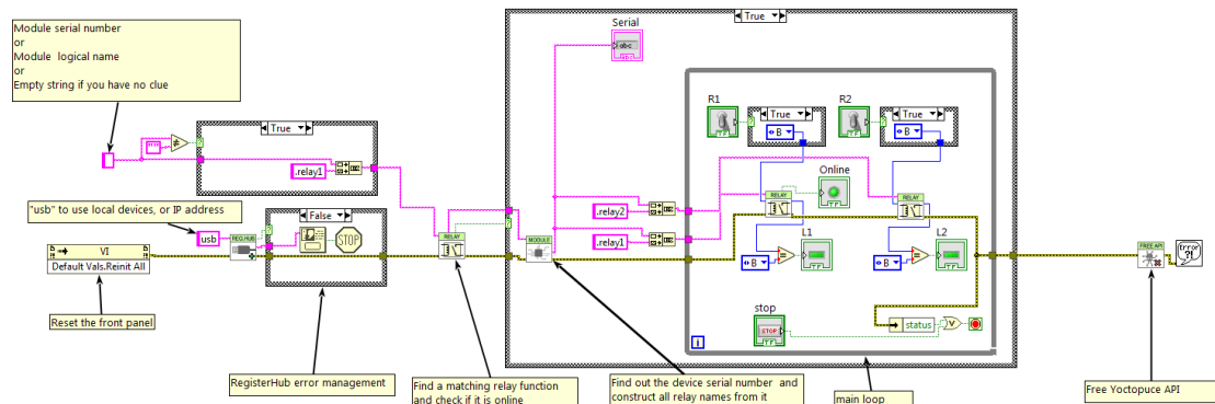
Exemple d'utilisation du Yocto-Relay dans LabVIEW
