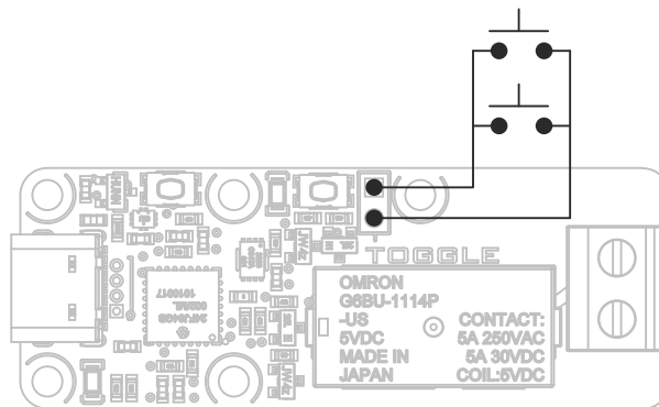
Câblage de boutons poussoirs pour commander le Yocto-LatchingRelay-C manuellement.
