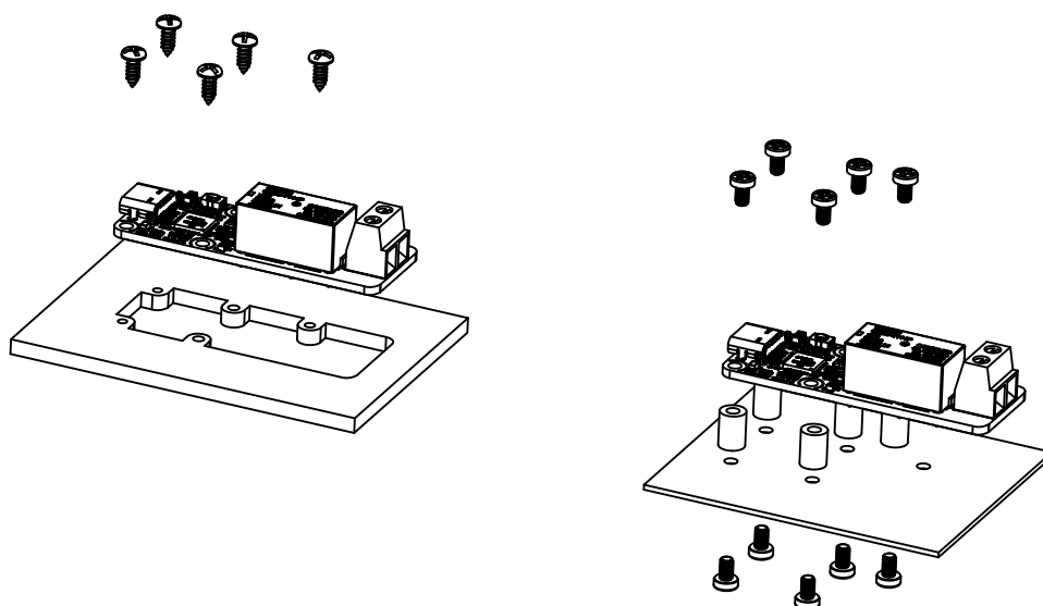
Exemples de montage sur un support.
