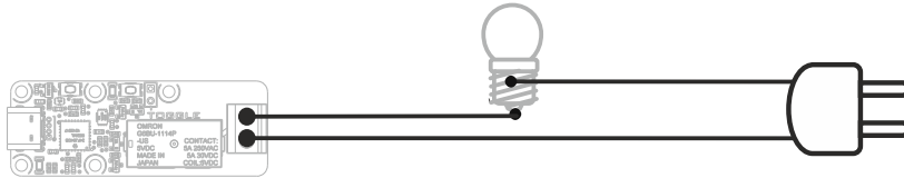
Commander une ampoule à l'aide de votre module Yocto-LatchingRelay-C.
