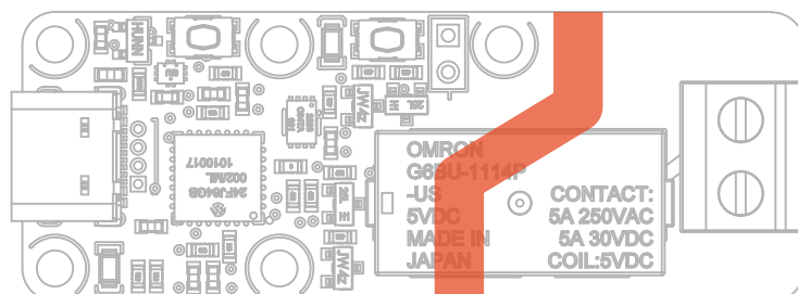
Barrière d'isolation de sécurité du module Yocto-LatchingRelay-C
