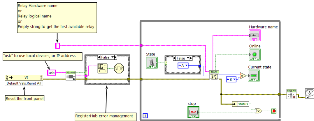
Exemple d'utilisation du Yocto-PowerRelay-V3 dans LabVIEW
