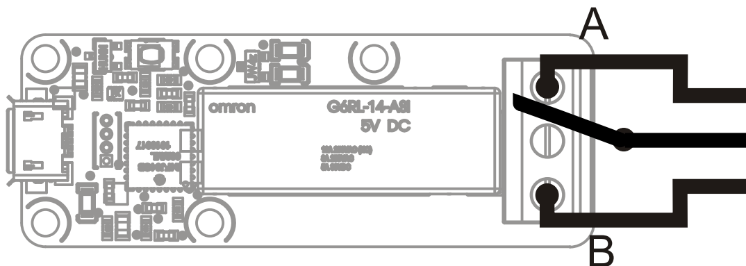
Câblage du relais à l'intérieur du module.
