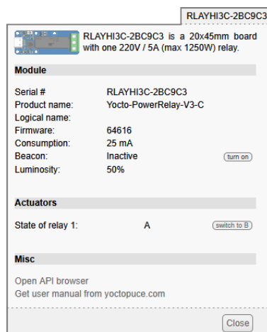
Propriétés du module Yocto-PowerRelay-V3-C.
