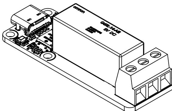
Le module Yocto-PowerRelay-V3-C
