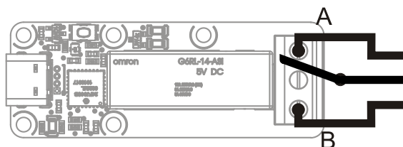
Câblage du relais à l'intérieur du module.
