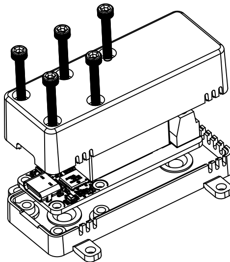
Vous pouvez installer votre Yocto-PowerRelay-V3-C dans un boîtier optionnel.
