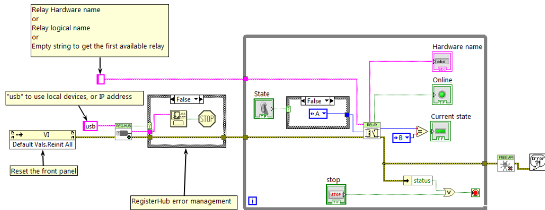
Exemple d'utilisation du Yocto-PowerRelay-V3-C dans LabVIEW
