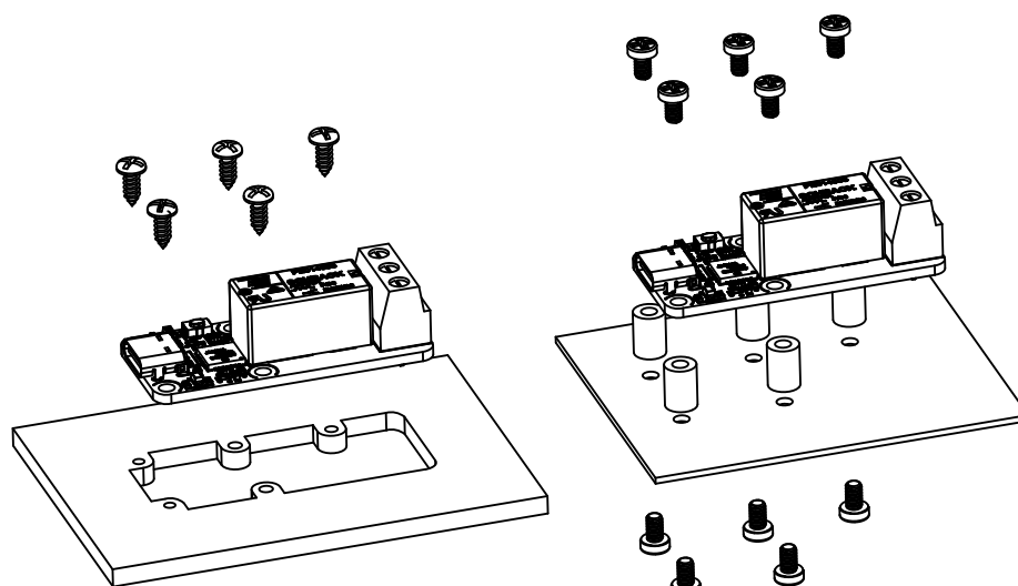
Exemples de montage sur un support.
