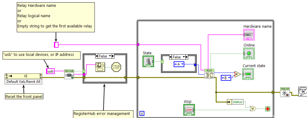
Exemple d'utilisation du Yocto-PowerRelay-V2-C dans LabVIEW
