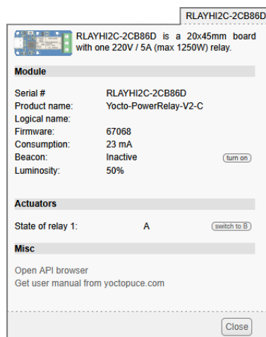
Propriétés du module Yocto-PowerRelay-V2-C.
