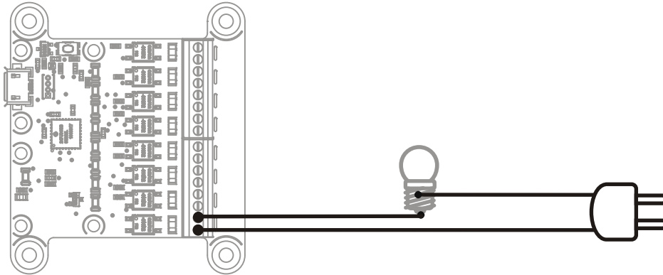
Commander une ampoule à l'aide de votre module Yocto-MaxiCoupler-V2.
