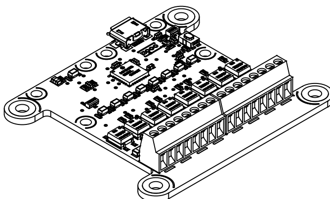
Le module Yocto-MaxiCoupler-V2
