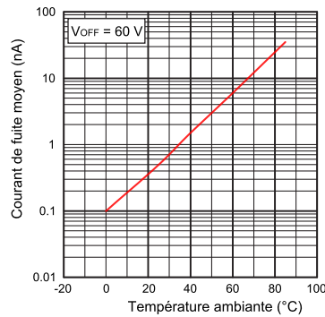
Courant de fuite moyen à 60V sur la plage de température étendue
