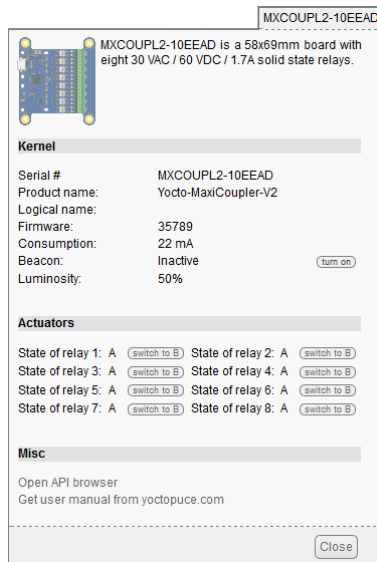
Propriétés du module Yocto-MaxiCoupler-V2.
