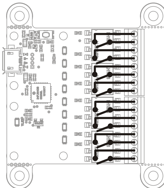
Câblage du relais à l'intérieur du module.
