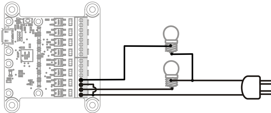
Commander deux ampoules à l'aide de votre module Yocto-MaxiCoupler-V2.
