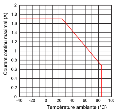
Courant de charge continu maximal toléré sur la plage de température étendue
