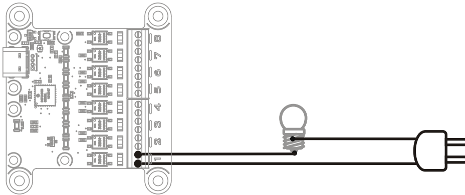
Commander une ampoule à l'aide de votre module Yocto-MaxiCoupler-V2-C.
