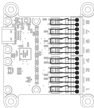
Câblage du relais à l'intérieur du module.
