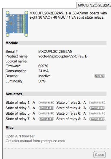
Propriétés du module Yocto-MaxiCoupler-V2-C.
