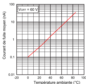
Courant de fuite moyen à 60V sur la plage de température étendue
