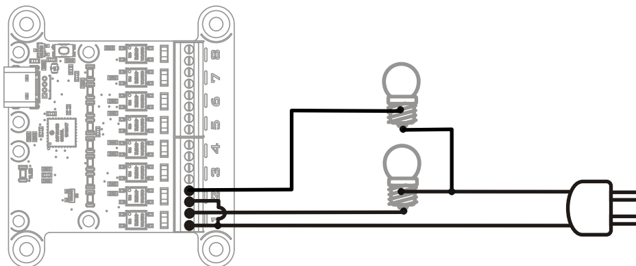
Commander deux ampoules à l'aide de votre module Yocto-MaxiCoupler-V2-C.
