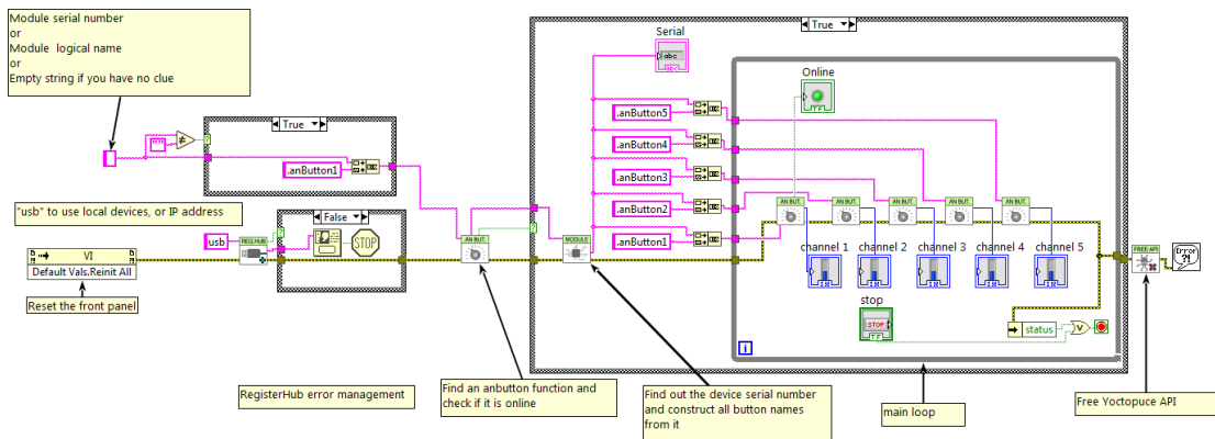
Exemple d'utilisation du Yocto-Knob-C dans LabVIEW
