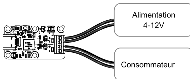
Câblage de l'alimentation commandée par le Yocto-WatchdogDC-C.
