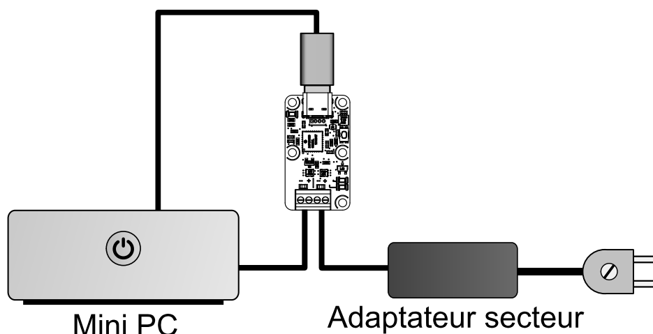
Utilisation typique du Yocto-WatchdogDC-C.
