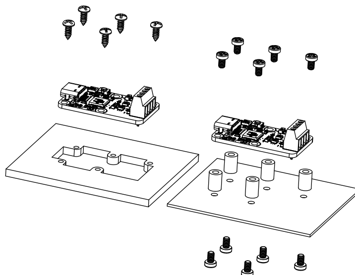
Exemples de montage sur un support.
