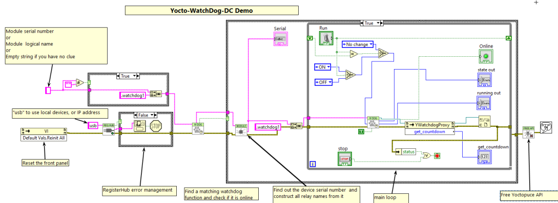
Exemple d'utilisation du Yocto-WatchdogDC-C dans LabVIEW
