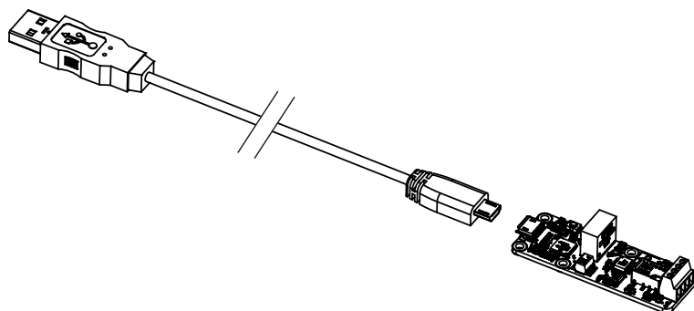
Vous devez raccorder votre module Yocto-PWM-Tx à l'aide d'un cable USB 2.0 de type A - micro B
