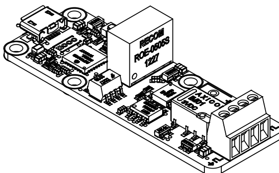
Le module Yocto-PWM-Tx
