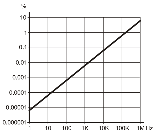
Corrélation entre la fréquence et la précision du duty-cycle.
