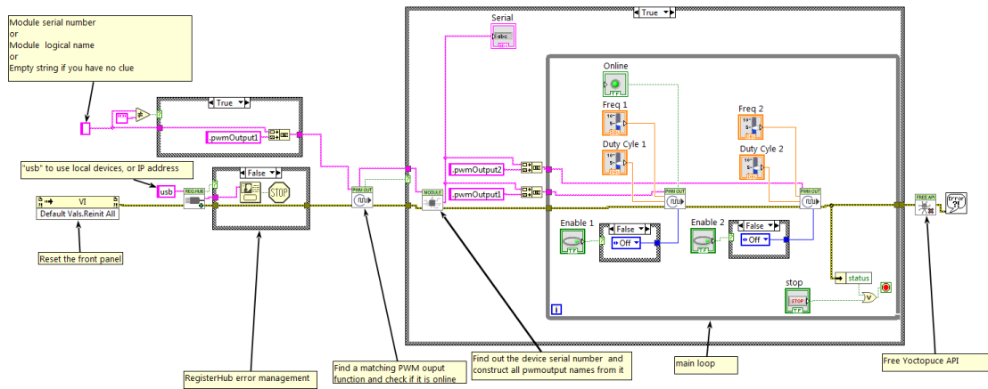
Exemple d'utilisation du Yocto-PWM-Tx-C dans LabVIEW
