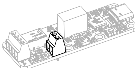
Utilisation d'un bornier pour l'alimentation externe.
