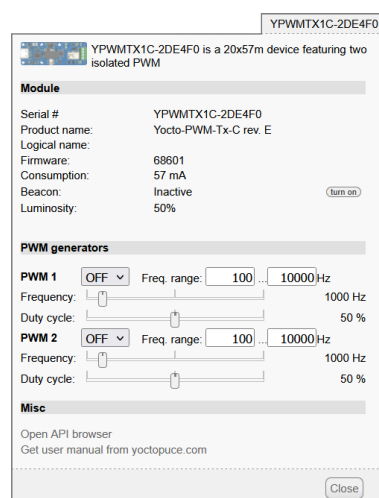
Propriétés du module Yocto-PWM-Tx-C.
