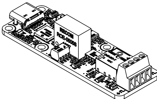
Le module Yocto-PWM-Tx-C
