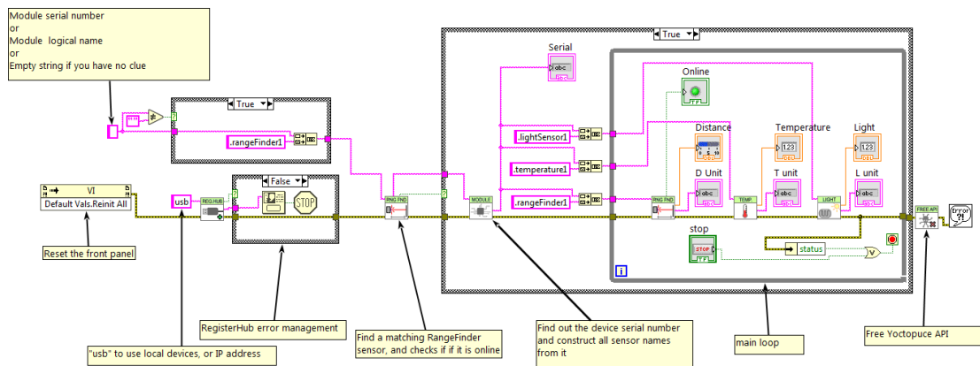
Exemple d'utilisation du Yocto-RangeFinder-C dans LabVIEW
