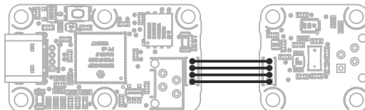
Câblage des sous-modules une fois ceux-ci séparés.
