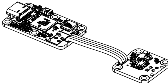
Déport du capteur à l'aide de simple câble nappe.
