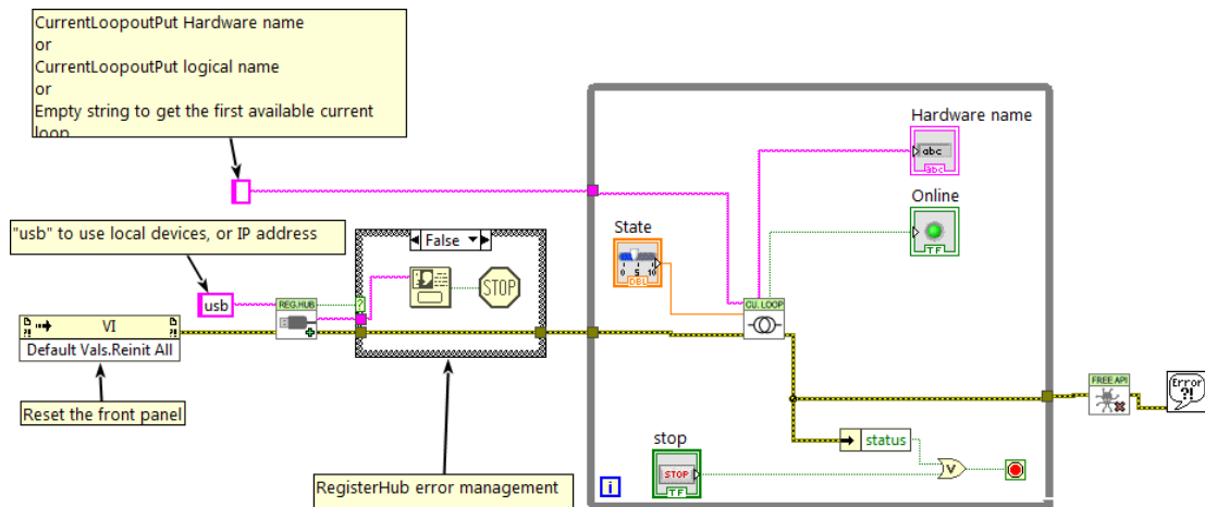
Exemple d'utilisation du Yocto-4-20mA-Tx dans LabVIEW
