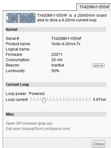
Propriétés du module Yocto-4-20mA-Tx.
