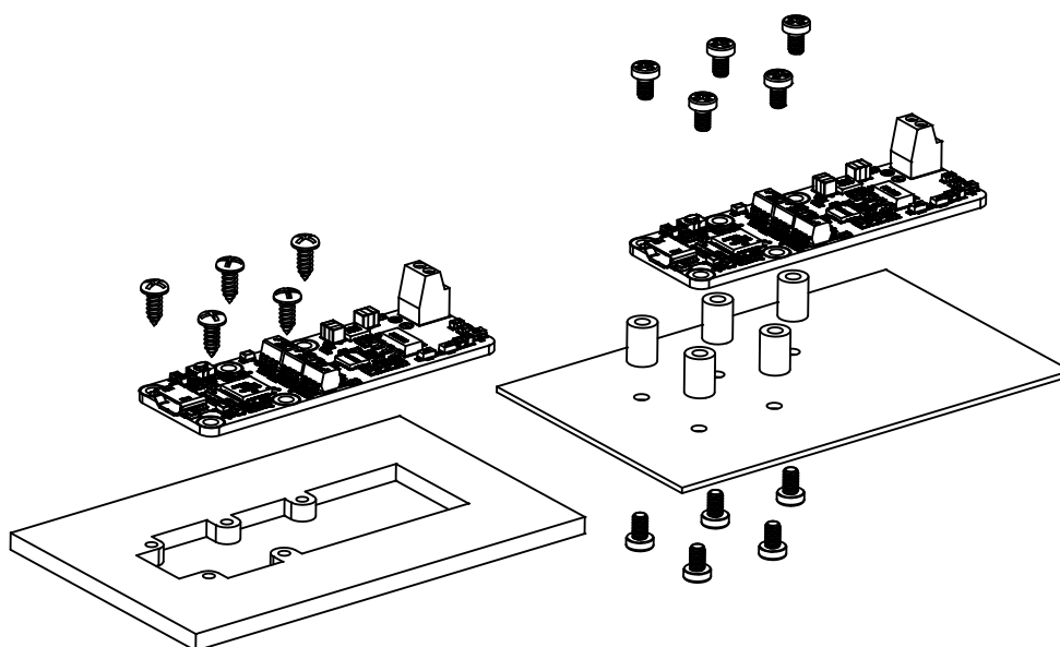
Exemples de montage sur un support.
