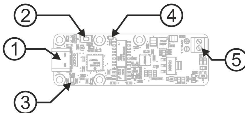
1: Prise USB-C 4: Indicateur de courant dans la boucle 2: Yocto-bouton 5: Connecteur de la boucle 3: Yocto-led
