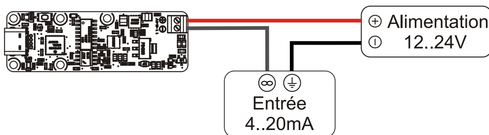
Câblage du Yocto-4-20mA-Tx-V2-C: le module régule le courant sur la boucle, qui est fourni par une alimentation externe.
