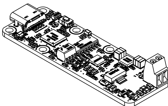
Le module Yocto-4-20mA-Tx-V2-C
