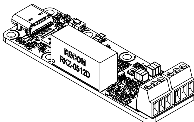
Le module Yocto-0-10V-Rx-C
