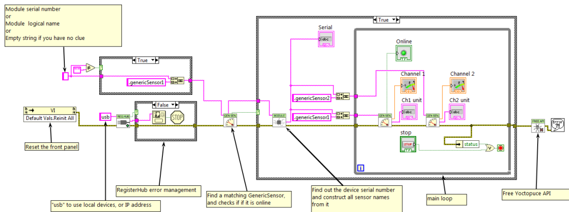
Exemple d'utilisation du Yocto-0-10V-Rx-C dans LabVIEW
