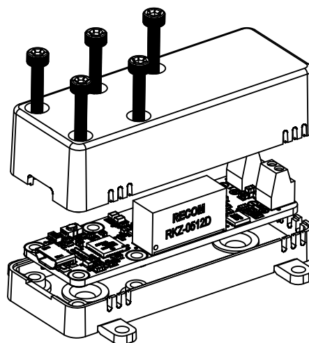
Vous pouvez installer votre Yocto-0-10V-Tx dans un boîtier optionnel.
