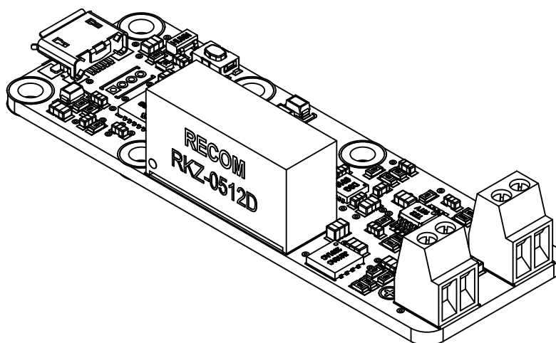
Le module Yocto-0-10V-Tx
