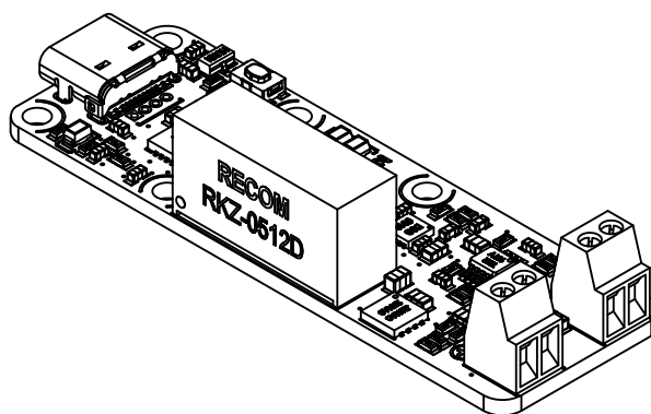
Le module Yocto-0-10V-Tx-C
