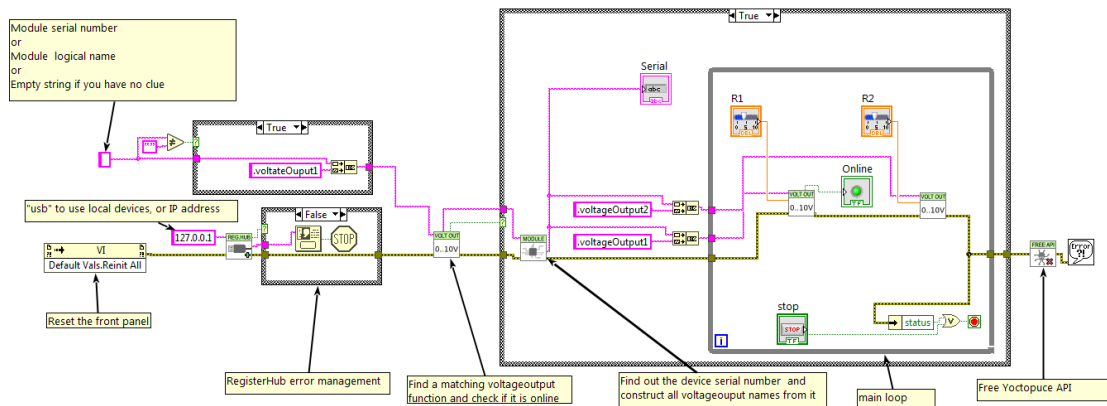
Exemple d'utilisation du Yocto-0-10V-Tx-C dans LabVIEW
