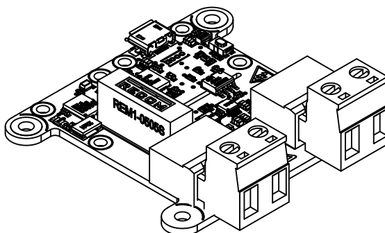
Le module Yocto-Watt
