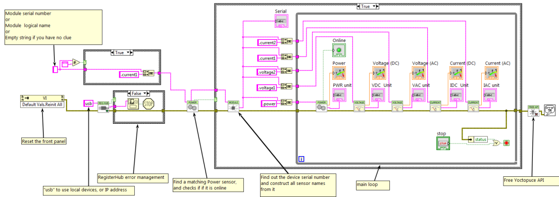
Exemple d'utilisation du Yocto-Watt dans LabVIEW
