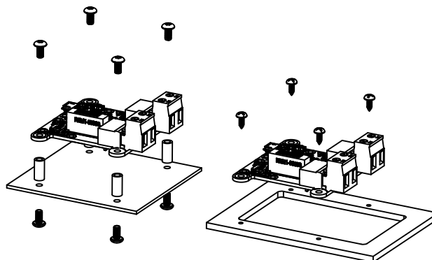
Exemples de montage sur un support.
