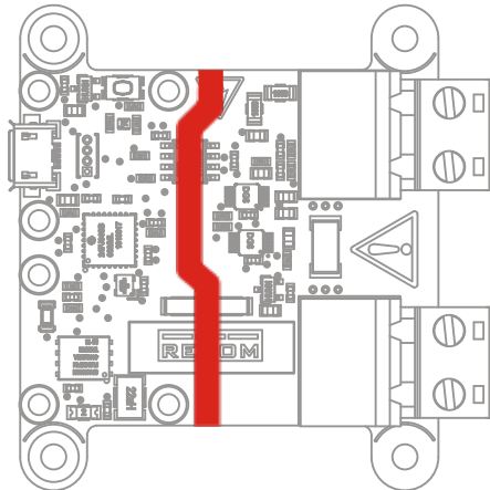
Barrière d'isolation de sécurité du module Yocto-Watt
