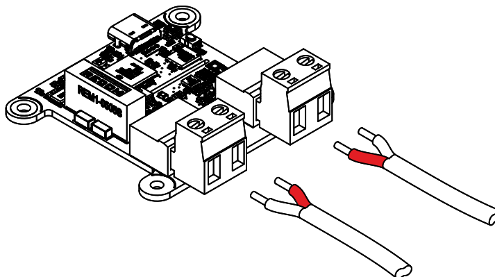
Les borniers se séparent en deux parties. Notez la symétrie de la polarité.
