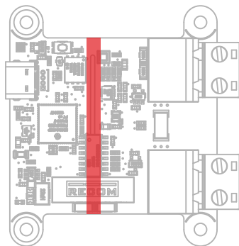
Barrière d'isolation de sécurité du module Yocto-Watt-V2-C
