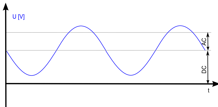
Tension alternative asymétrique. C'est la somme d'une tension continue et une tension alternative.
