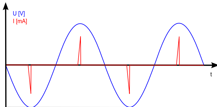
Exemple de profil de consommation pour une charge avec distorsion harmonique.
