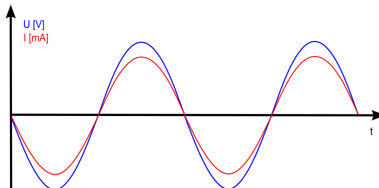
Profil de consommation d'une charge purement résistive alimentée sur le secteur.
