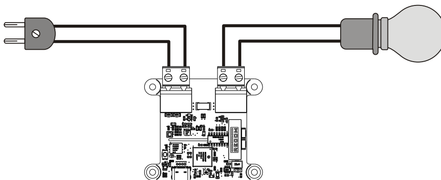
Le Yocto-Watt-V2-C doit être intercalé entre la source et le consommateur.
