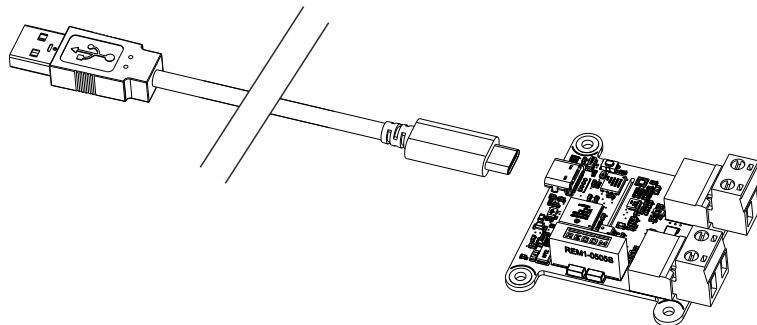
Vous devez raccorder votre module Yocto-Watt-V2-C à l'aide d'un cable USB 2.0 de type A - Type-C
