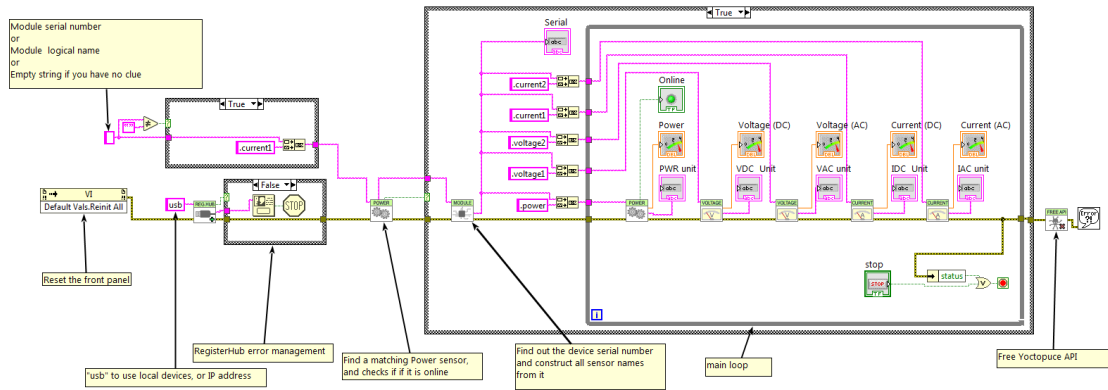
Exemple d'utilisation du Yocto-Watt-V2-C dans LabVIEW
