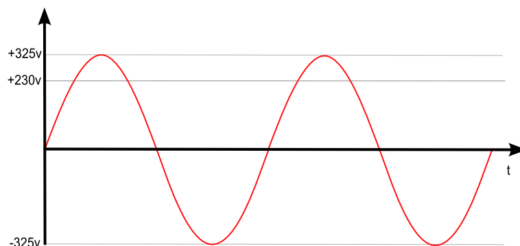
Tension alternative, par exemple la tension du secteur en Europe: elle change de manière périodique.
