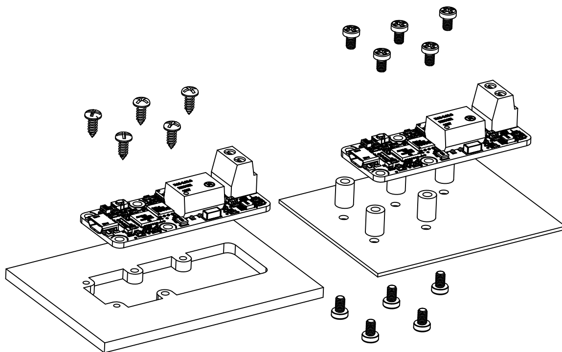
Exemples de montage sur un support.
