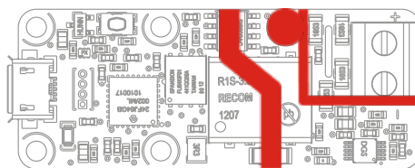
Barrière d'isolation de sécurité du module Yocto-Volt
