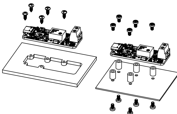
Exemples de montage sur un support.
