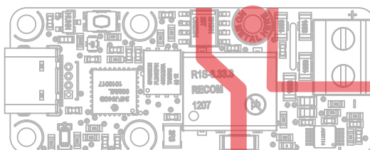
Barrière d'isolation de sécurité du module Yocto-Volt-C
