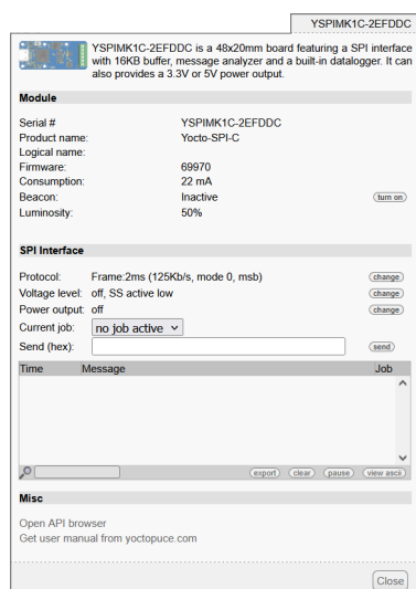
Propriétés du module Yocto-SPI-C.
