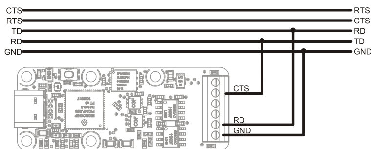
Câblage pour utiliser le Yocto-Serial-C en mode analyseur.
