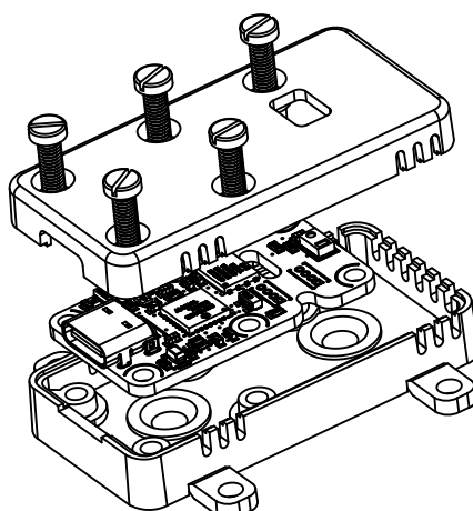
Vous pouvez installer votre Yocto-Proximity-C dans un boîtier optionnel.
