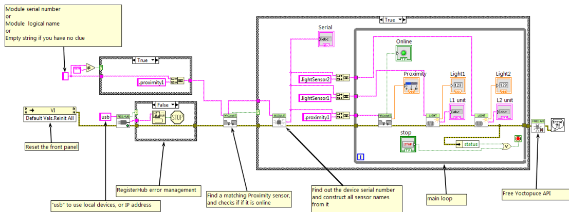
Exemple d'utilisation du Yocto-Proximity-C dans LabVIEW
