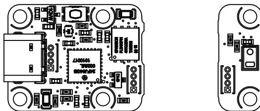
Le module Yocto-Proximity-C est conçu pour pouvoir être séparé en deux parties...
