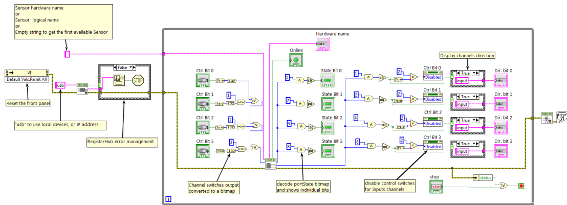
Exemple d'utilisation du Yocto-IO dans LabVIEW
