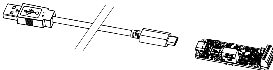
Vous devez raccorder votre module Yocto-IO-V2-C à l'aide d'un câble USB 2.0 de type A - USB-C
