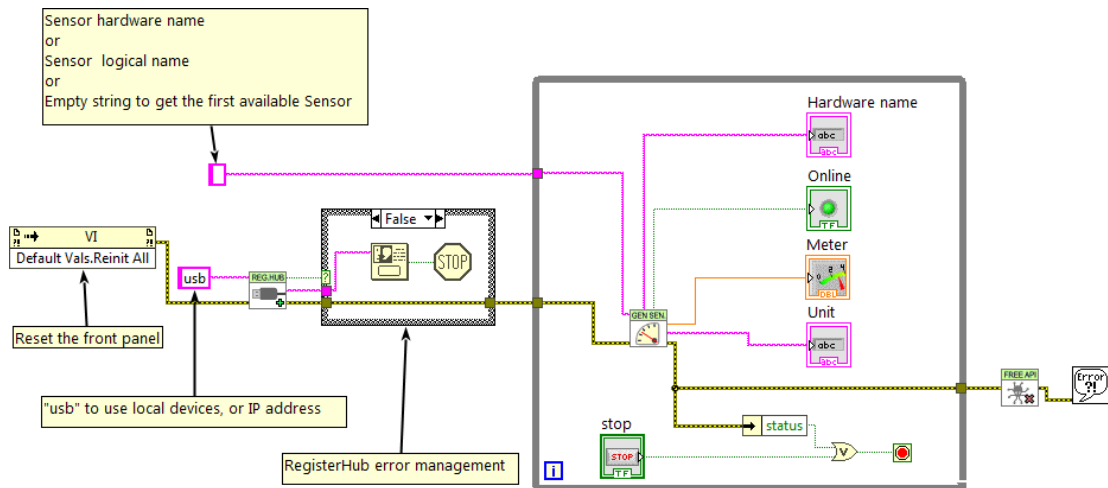
Exemple d'utilisation du Yocto-milliVolt-Rx-C dans LabVIEW
