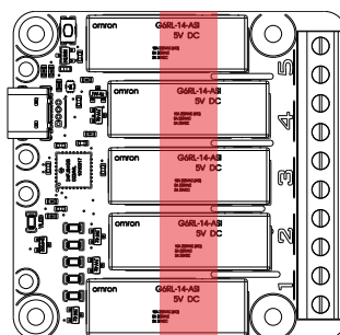
Barrière d'isolation de sécurité du module Yocto-MaxiPowerRelay-C
