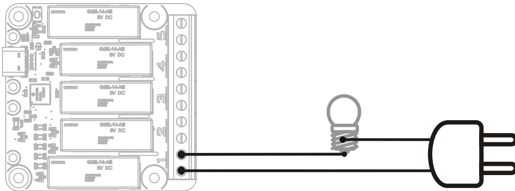
Commander une ampoule à l'aide de votre module Yocto-MaxiPowerRelay-C.
