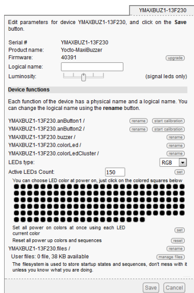
Configuration du module Yocto-MaxiBuzzer.
