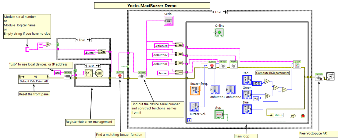
Exemple d'utilisation du Yocto-MaxiBuzzer dans LabVIEW
