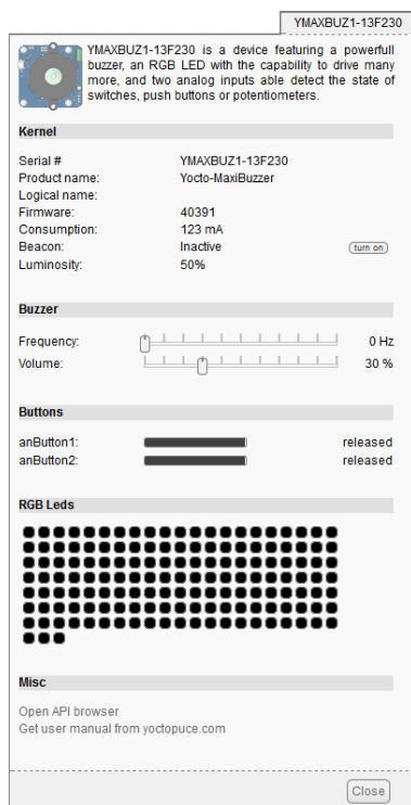
Propriétés du module Yocto-MaxiBuzzer.
