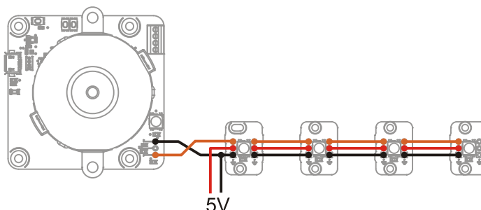
Câblage avec une alimentation externe
