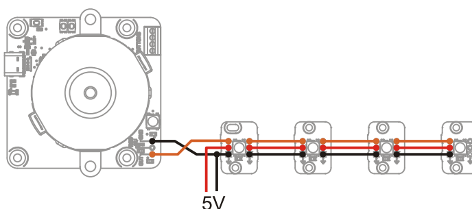
Câblage avec une alimentation externe
