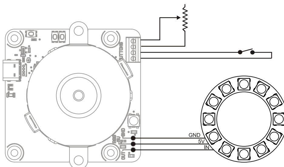
Exemple de câblage d'un bouton poussoir et d'un potentiomètre et de LED supplémentaires
