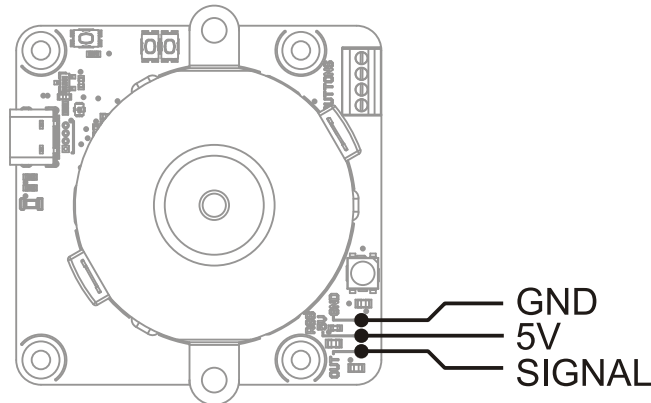
Le module Yocto-MaxiBuzzer-C dispose d'une sortie pour piloter des LED supplémentaires.
