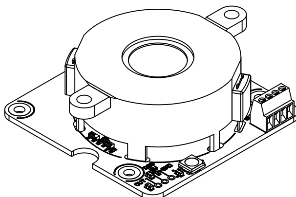
Le module Yocto-MaxiBuzzer-C
