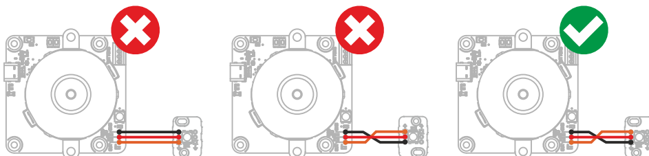
Attention à la polarité et au sens de LEDs, chacune a une entrée et une sortie.
