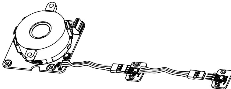
Exemple de câblage des sous-modules à l'aide de câbles de servos.
