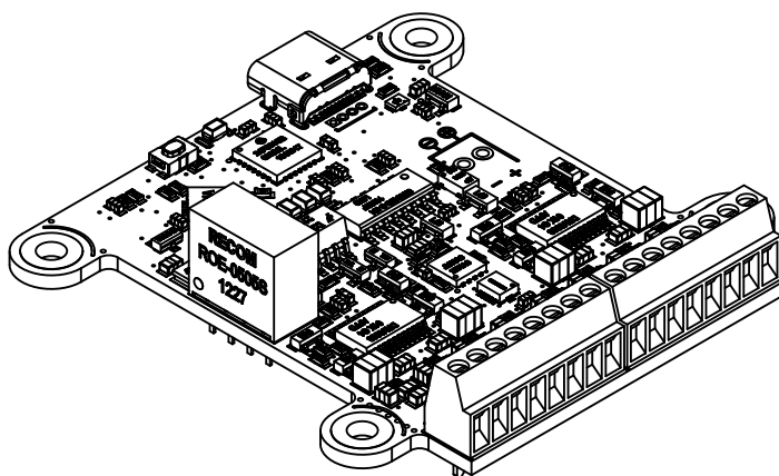
Le module Yocto-Maxi-IO-V3-C
