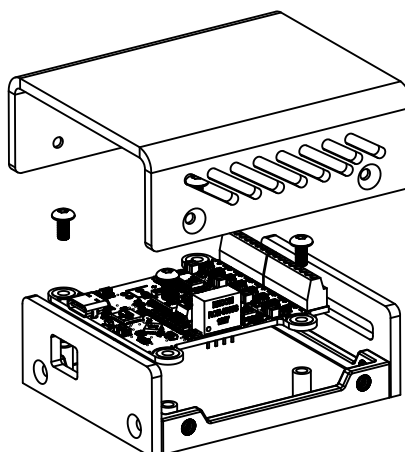
Vous pouvez installer votre Yocto-Maxi-IO-V3-C dans un boîtier optionnel.
