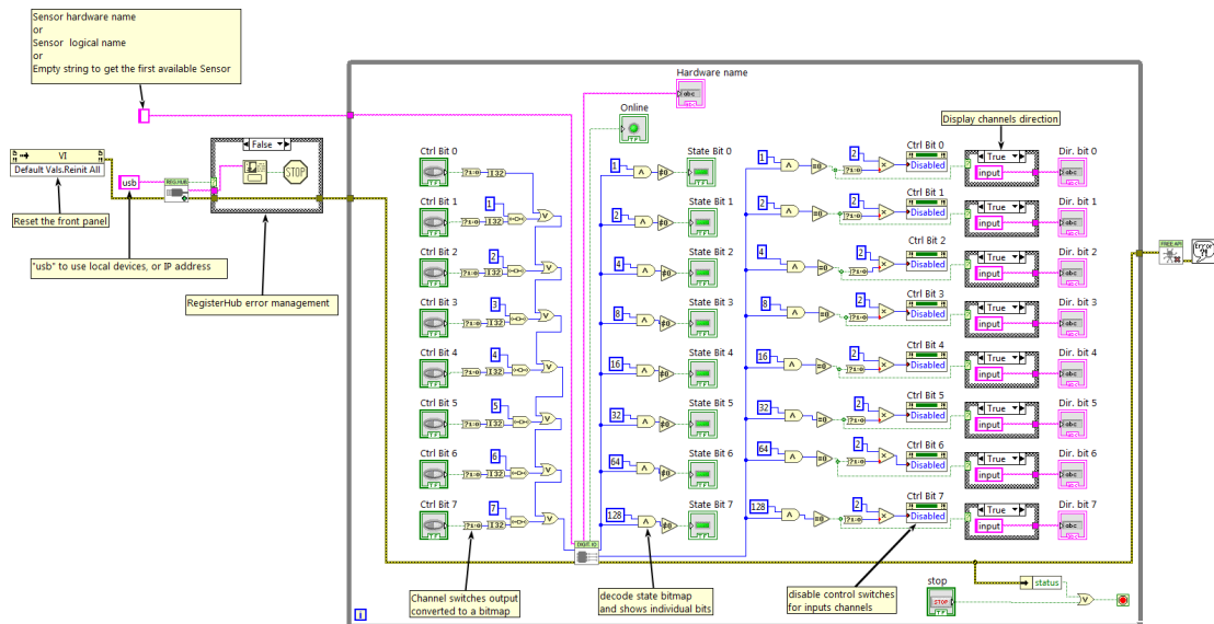
Exemple d'utilisation du Yocto-Maxi-IO-V3-C dans LabVIEW
