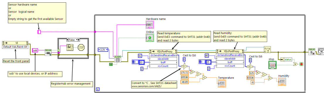
Lire un capteur Sensirion SHT25 avec un Yocto-I2C
