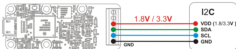
Connexion avec une interface I2C 1.8V ou 3.3V
