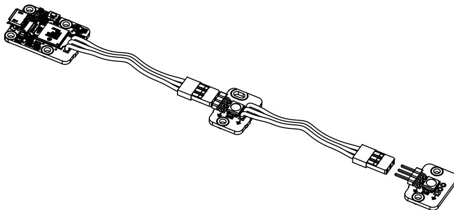
Exemple de câblage des sous-modules à l'aide de câbles de servos.
