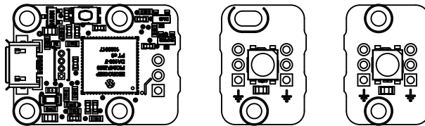
Le module Yocto-Color-V2 est conçu pour pouvoir être séparé en trois parties.
