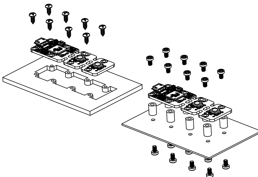
Exemples de montage sur un support.
