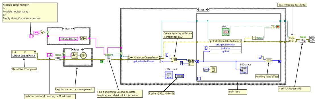
Exemple d'utilisation du Yocto-Color-V2 dans LabVIEW
