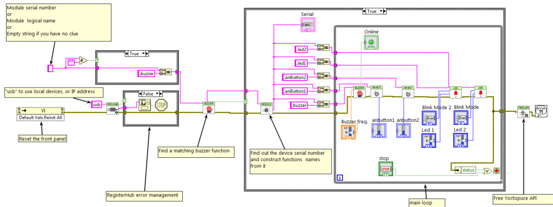
Exemple d'utilisation du Yocto-Buzzer-C dans LabVIEW
