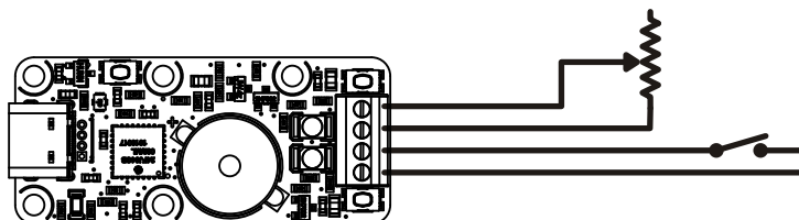
Exemple de câblage d'un bouton poussoir et d'un potentiomètre.
