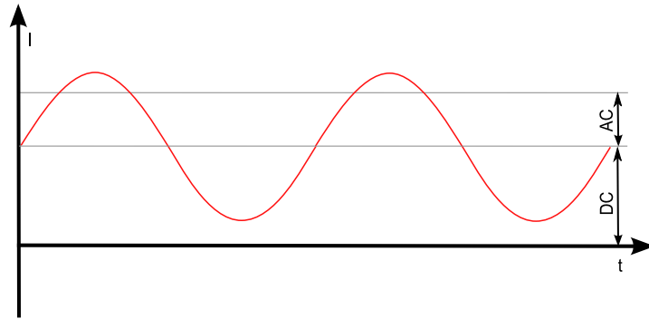
Courant alternatif asymétrique. C'est la somme d'un courant continu et d'un courant alternatif.
