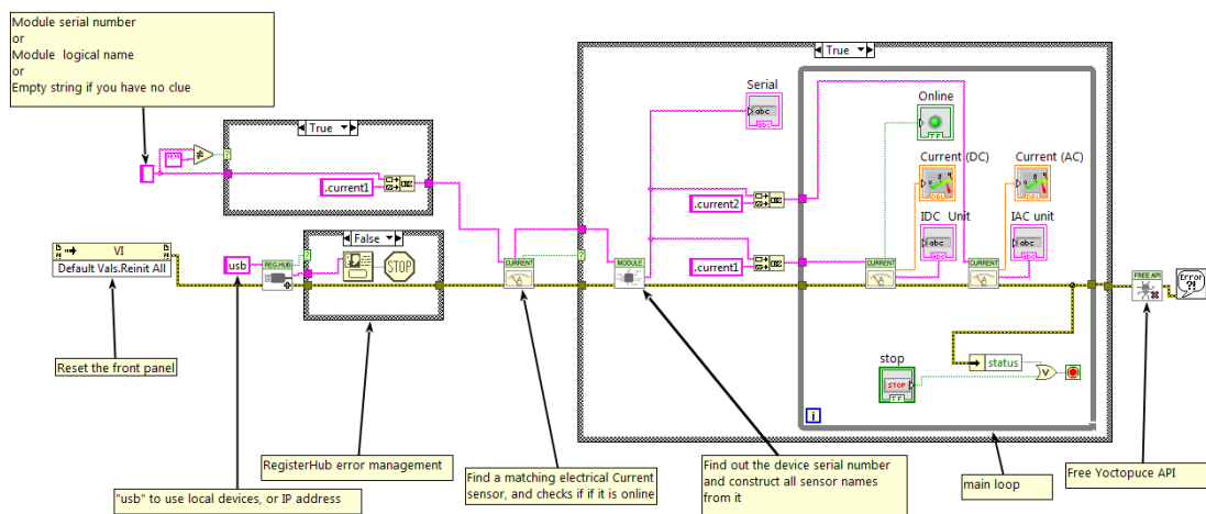
Exemple d'utilisation du Yocto-Amp-C dans LabVIEW
