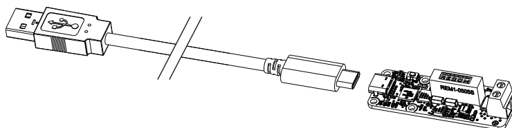
Vous devez raccorder votre module Yocto-Amp-C à l'aide d'un câble USB 2.0 de type A - USB-C
