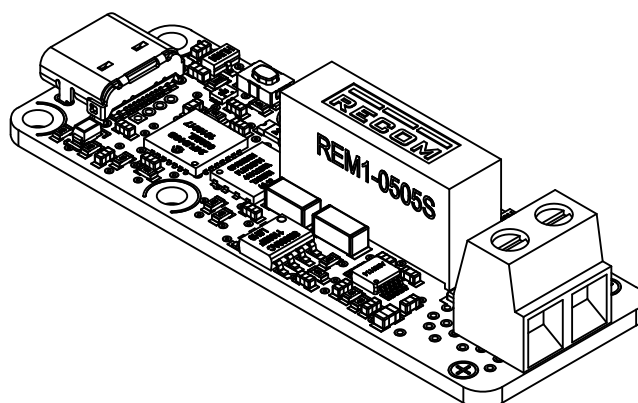
Le module Yocto-Amp-C
