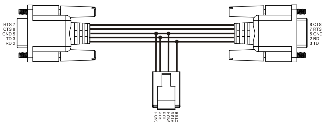
Câblage pour utiliser le Yocto-RS232-C en mode analyseur.
