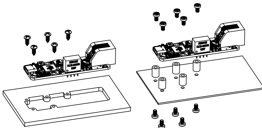
Exemples de montage sur un support.
