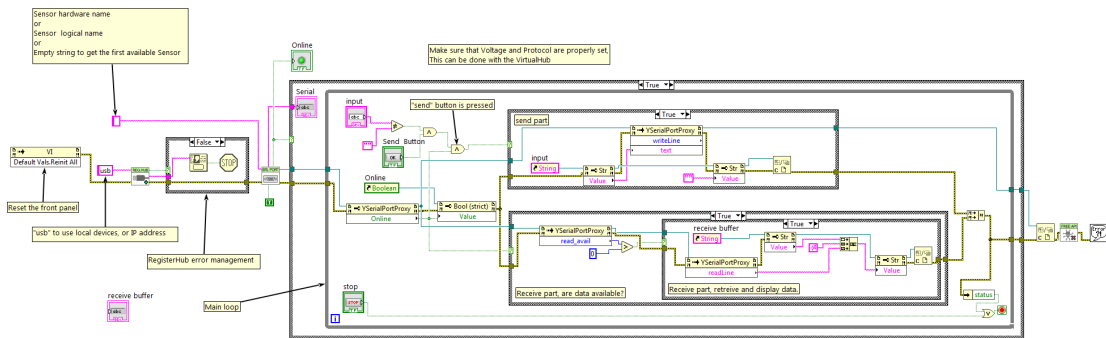
Exemple d'utilisation du Yocto-RS232-C dans LabVIEW
