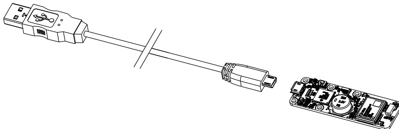
Vous devez raccorder votre module Yocto-GPS-V2 à l'aide d'un câble USB 2.0 de type A - micro B
