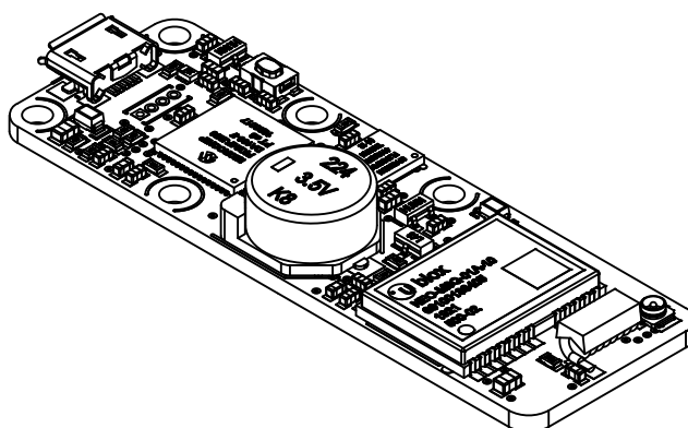
Le module Yocto-GPS-V2
