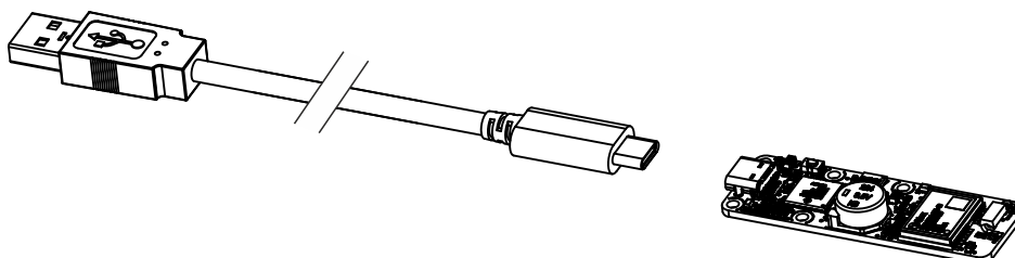
Vous devez raccorder votre module Yocto-GPS-V2-C à l'aide d'un cable USB 2.0 de type A - USB-C
